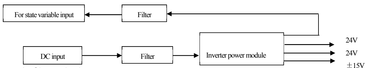
Figure2—5 Powermodul
